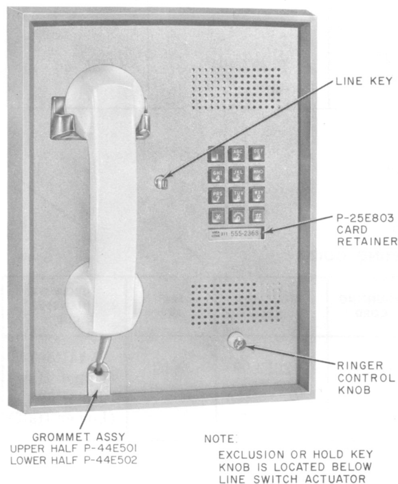
Fig. 1—2751-Type Telephone Set
