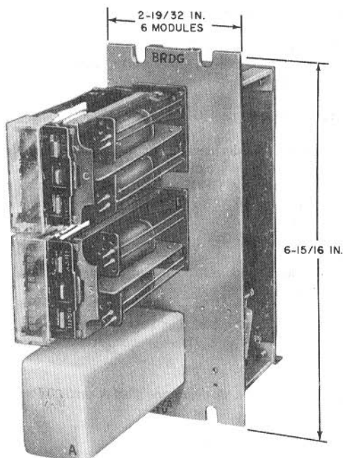
Fig. 1—237B Key Telephone Unit
