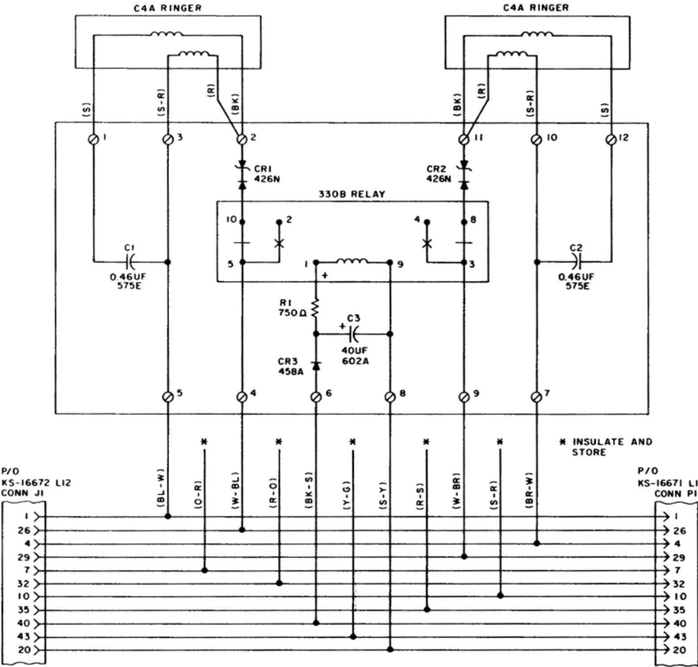
Fig. 29—Schematic, 24A Apparatus Unit
