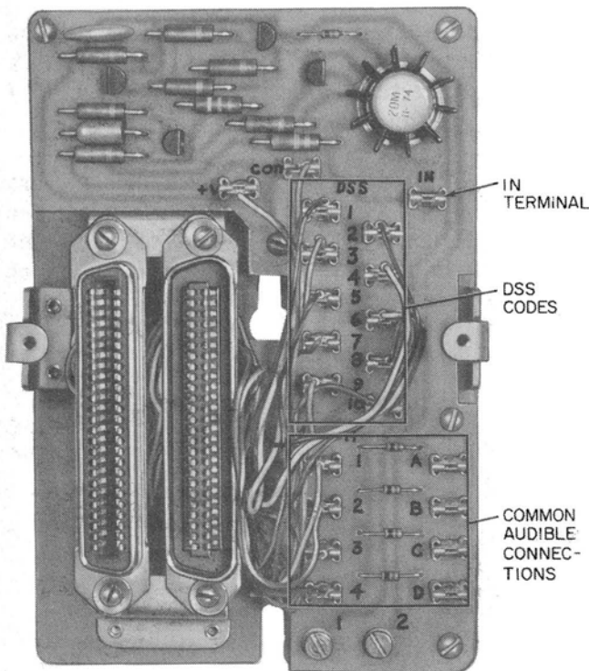
Fig. 17—25A Apparatus Unit Base
