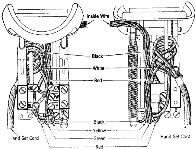
Fig. 4—213E Type Hand Telephone Sets.
