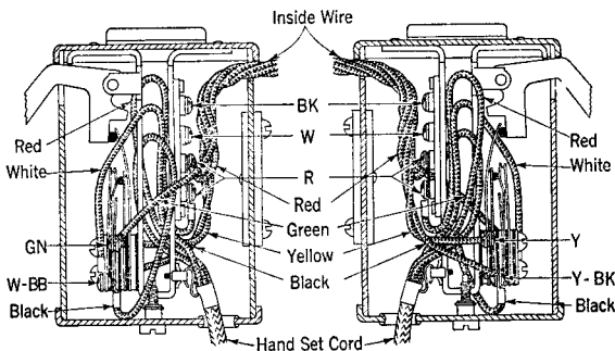
Fig. 1—201A Type Hand Telephone Sets.
