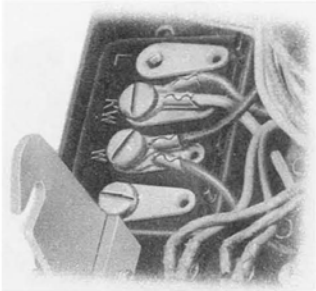
Fig. 5—Auxiliary Terminal Block (P-16A368)
