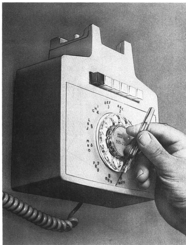
Fig. 20—Installing 851A (MD) or 852A Faceplate
