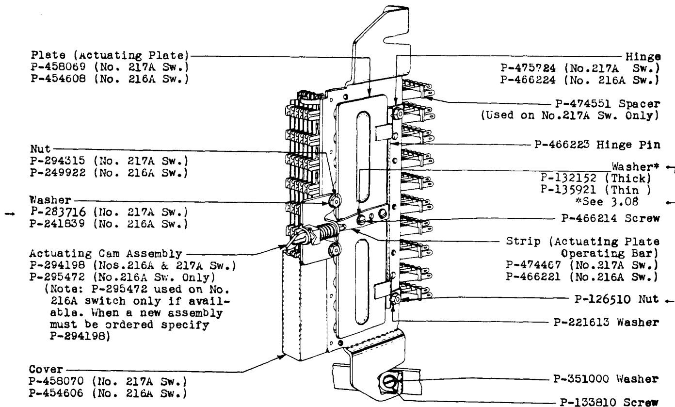
Fig. 1 - Nos. 216A and 217A Switches
