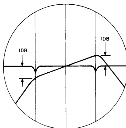
A. NO TERMINATION SLOPE CKT OFF
