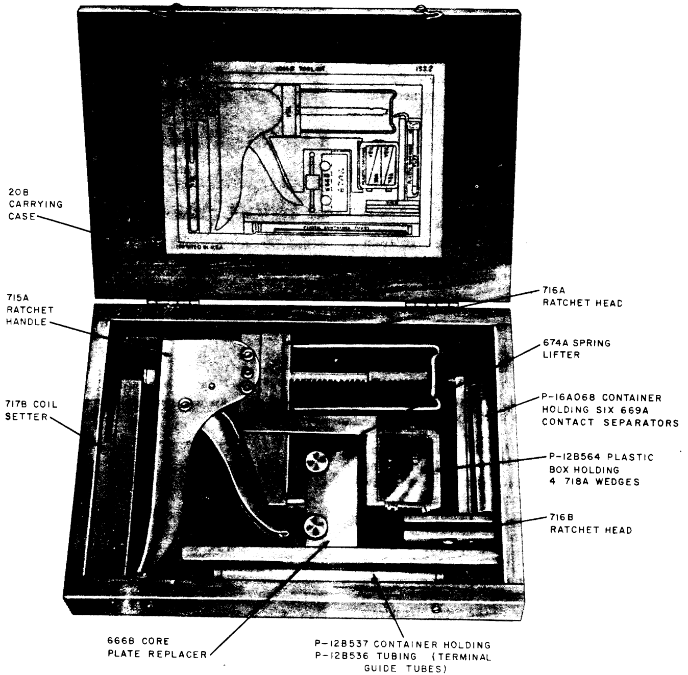
Fig. 24—1014B Tool Kit
