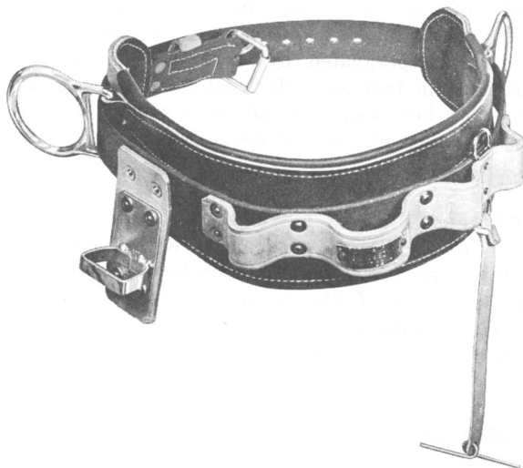
Fig. 2—D Body Belt
