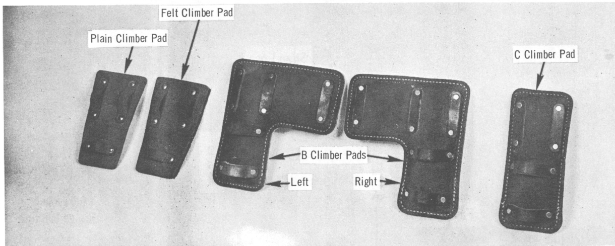
Fig. 4 — Pads
