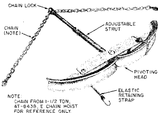
Fig. 3—G Slack Puller
