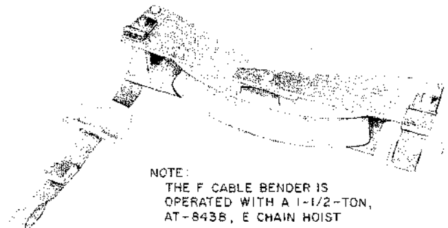
Fig. 1—F Cable Bender
