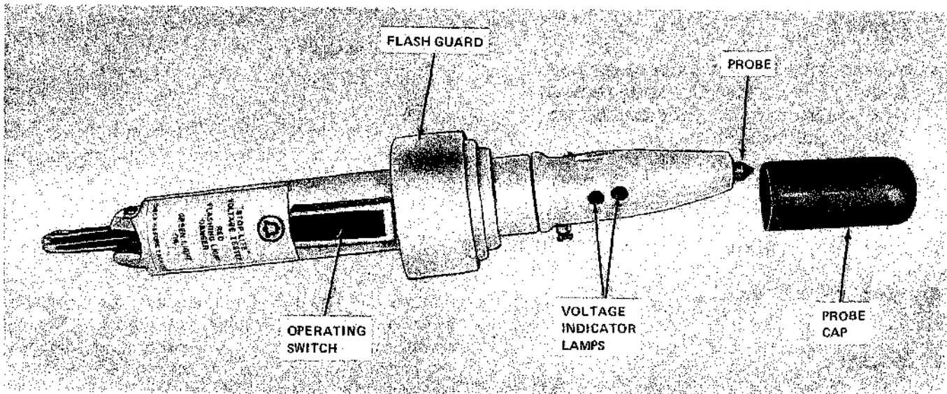
Fig. 1—188A Test Set
