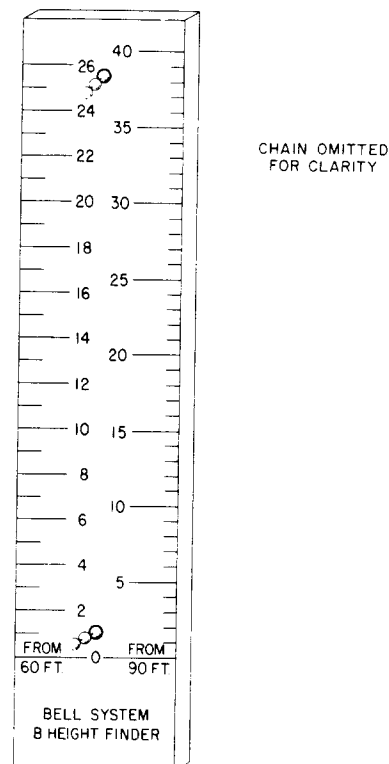
Fig. 6—B Height Finder
