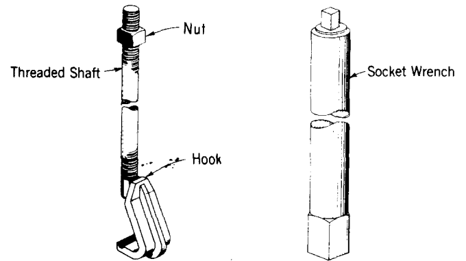
Fig. 15—E Strand Shifter
