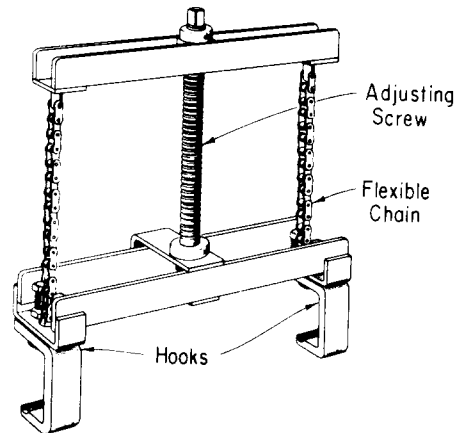
Fig. 13—D Strand Shifter
