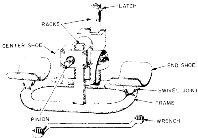
Fig. 2—E Cable Bender
