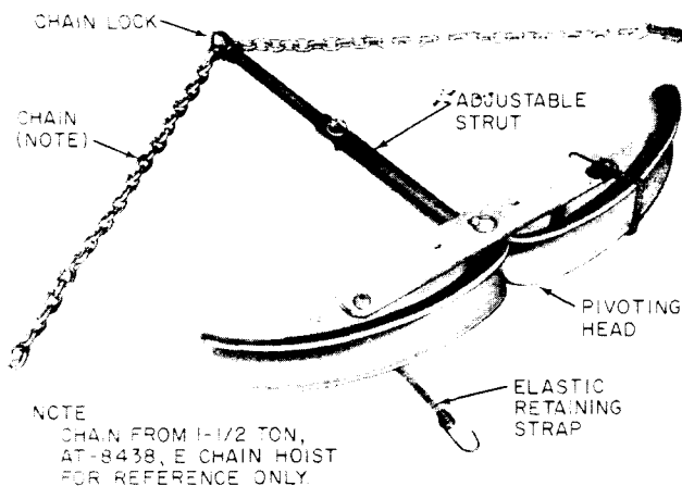
Fig. 3—G Slack Puller
