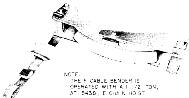
Fig. 1—F Cable Bender
