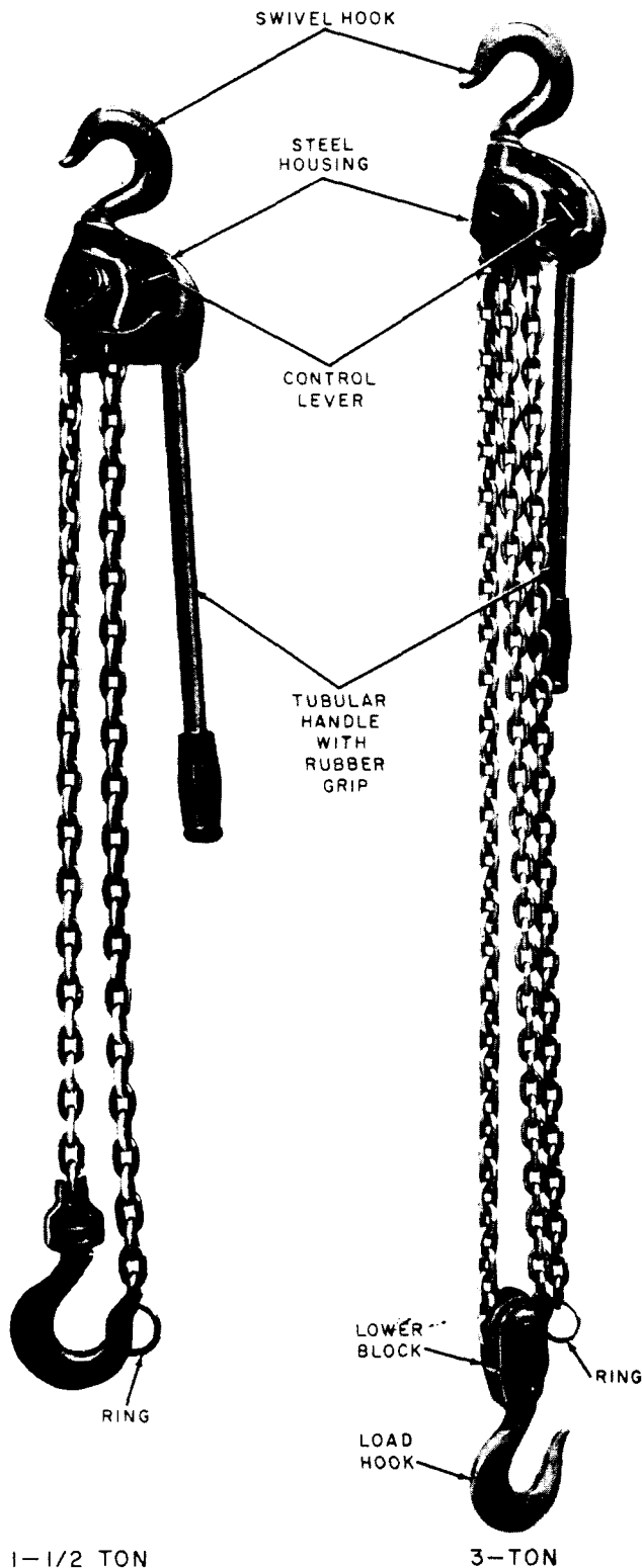
Fig. 1—E Chain Hoist
