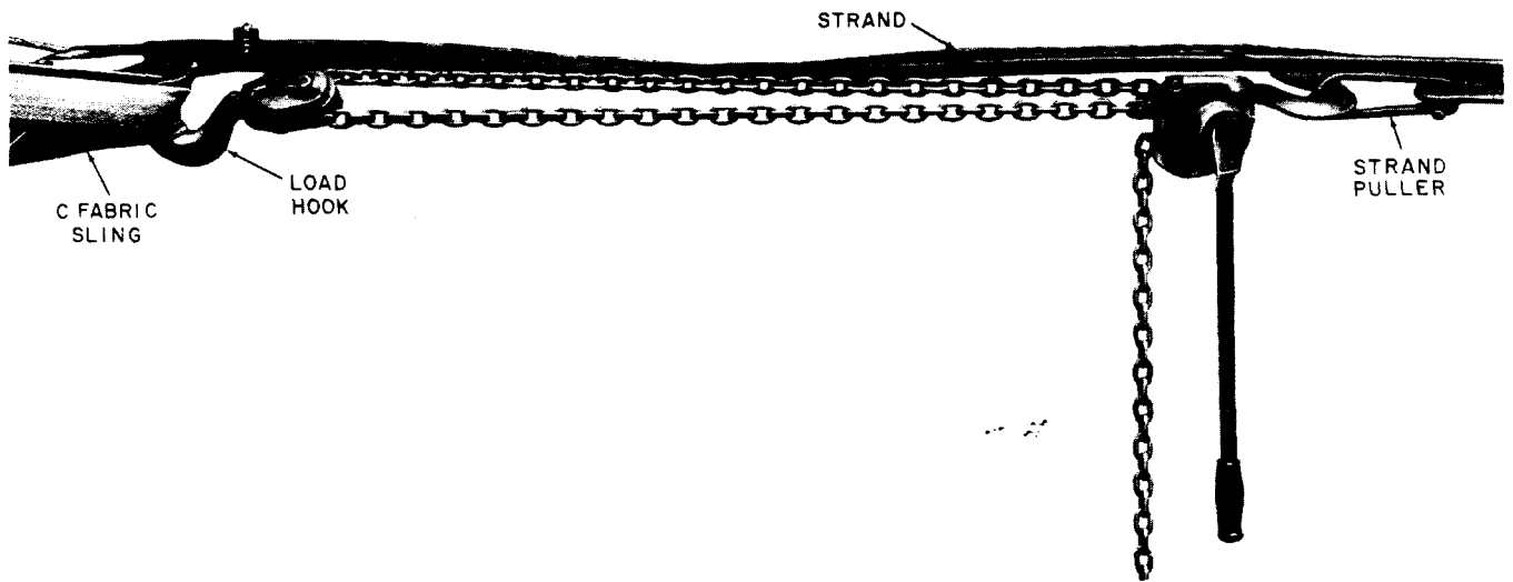
Fig. 5—Horizontal Position
