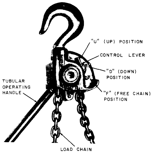
Fig. 3—Control Lever
