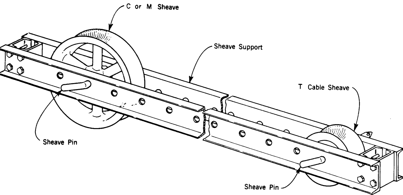
Fig. 1—Pulling Frame
