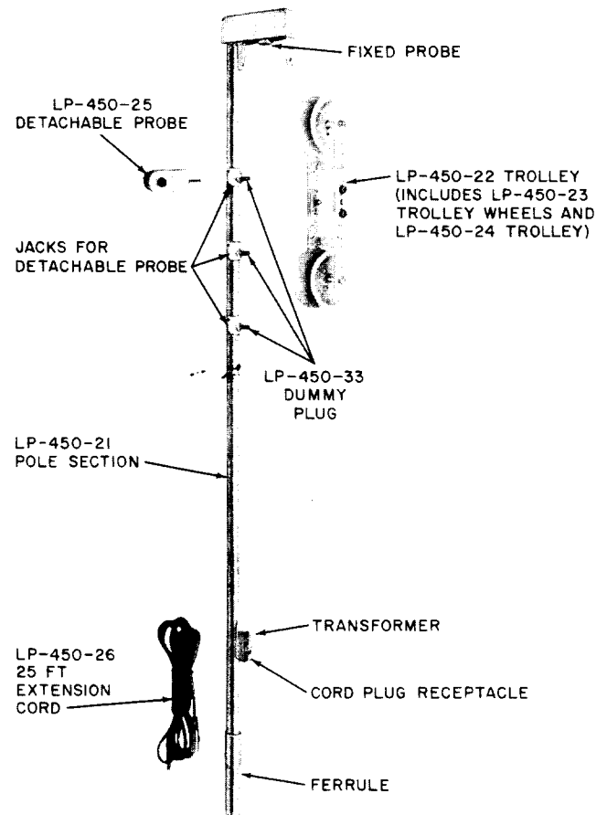
Fig. 11—Lumidor LP-455 Pole Probe
