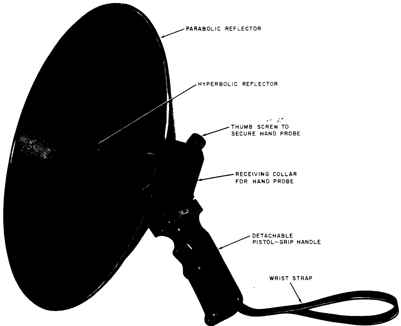
Fig. 14—B Ultrasonic Reflector
