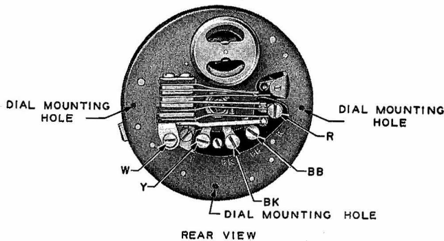
FIG. 4—5H-TYPE DIAL
