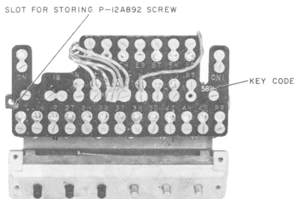
Fig. 7—589-Type Key, Top
