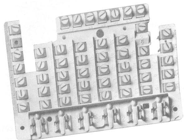
Fig. 6—636A Key, Top
