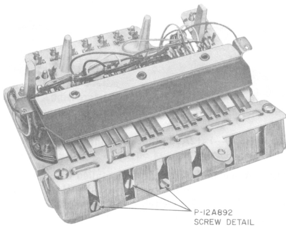
Fig. 4—636A Key, Bottom
