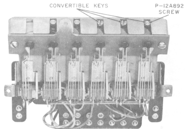
Fig. 5—589-Type Key, Bottom
