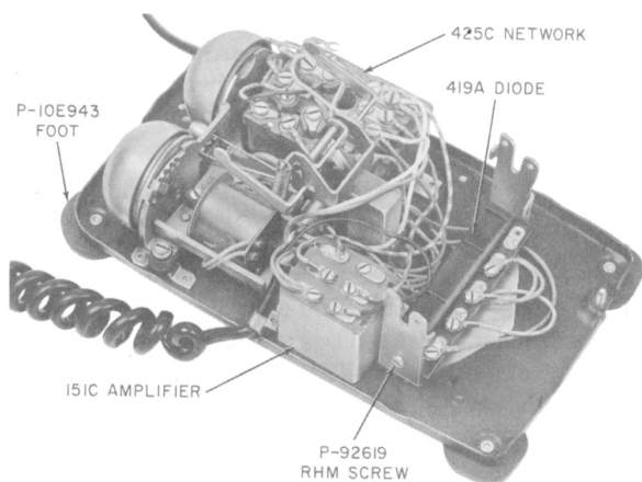
Fig. 2—507-Type Set, Interior
