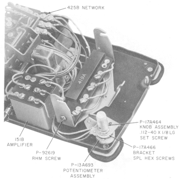
Fig. 8—532-Type Set, Interior
