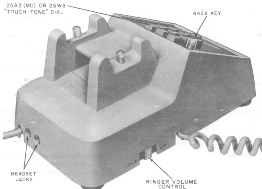
Fig. 1—1514B Telephone Set
