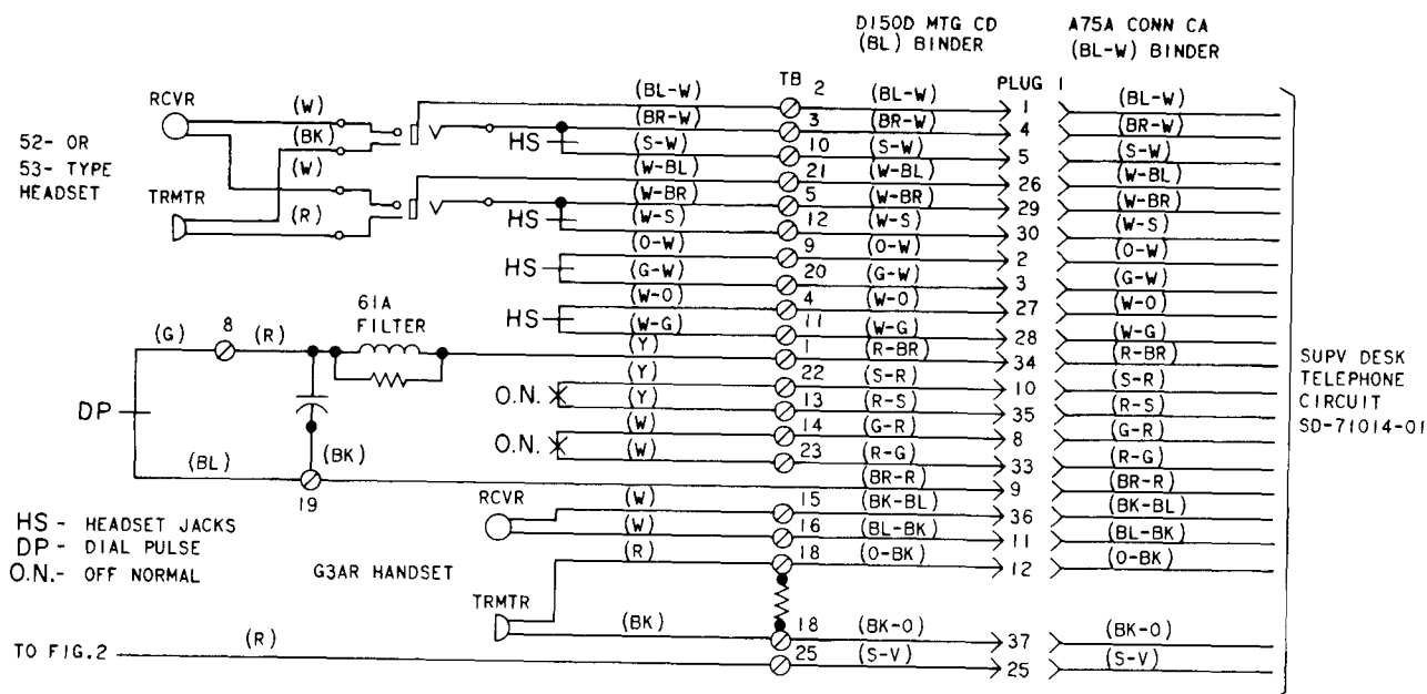
A. 609BI TELEPHONE SET
