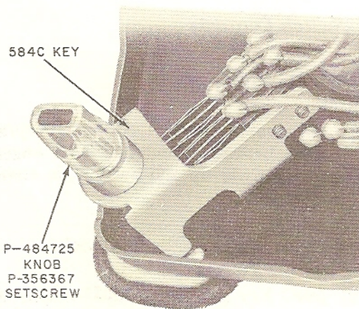
Fig. 27 — 584C Key
