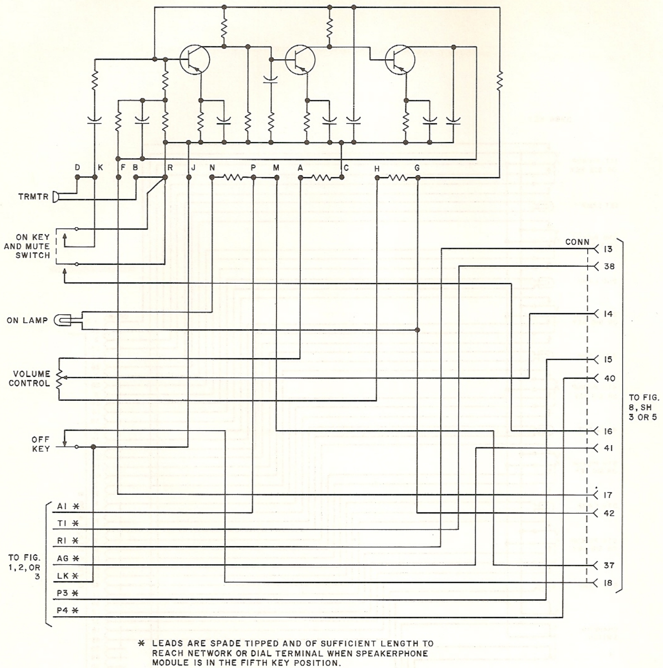
Fig. 6—667B Transmitter
