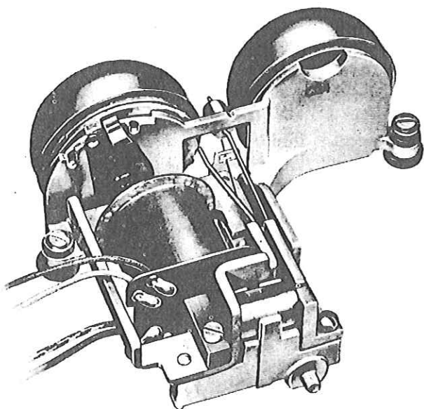
Fig. 12—C2A Ringer
