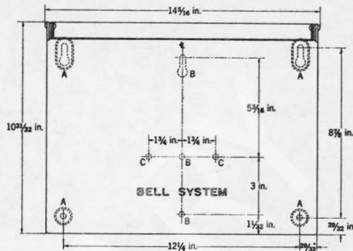
FIG. 4—159A BACKBOARD
