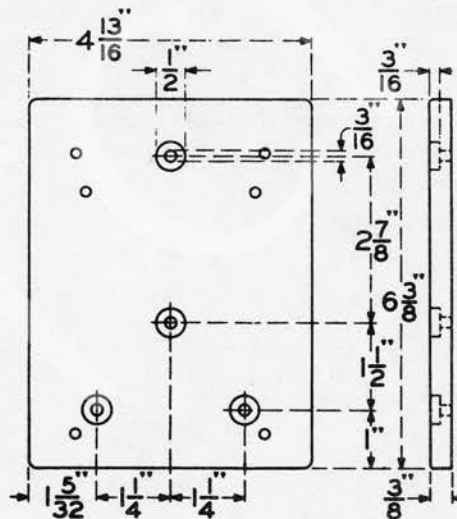
FIG. 1—171A BACKBOARD
